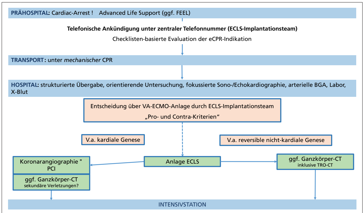
Abb. 1: eCPR-Algorithmus
